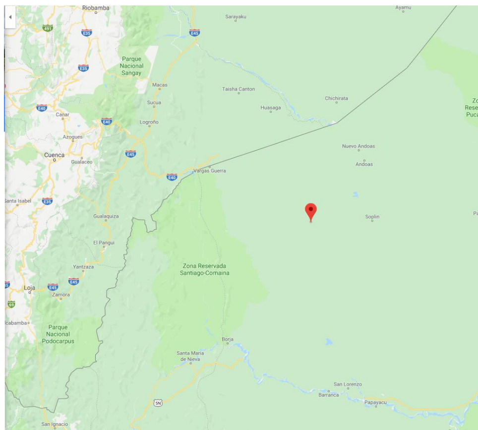
Figura 1. Localización del evento del día de hoy 18/01/2019, a las 16h26 con una magnitud de 5.9
