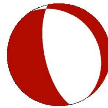
Figura 2. Mecanismo focal de tipo normal del evento del 01-06-2016 a las 05h05 (TL)
