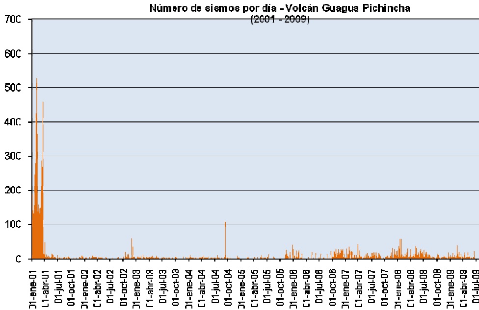
Fig. 1 Numero de sismos por día registrados en la estación CGGP.
