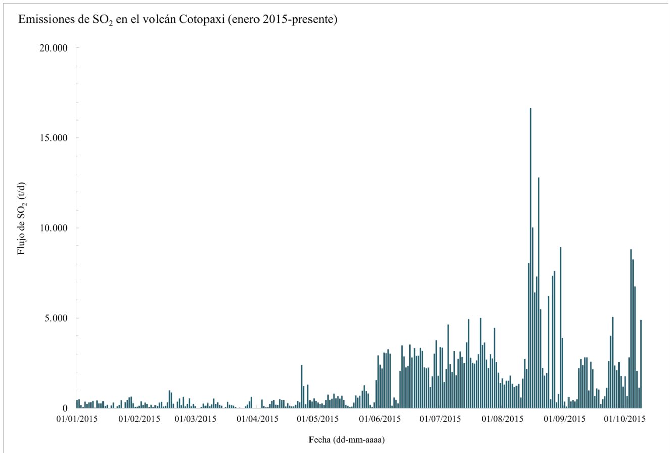
Fig. 2. Representación del máximo promedio diario flujo de SO_2 entre todas las estaciones del volcán Cotopaxi desde enero 2015 al 9 de octubre del 2015.
