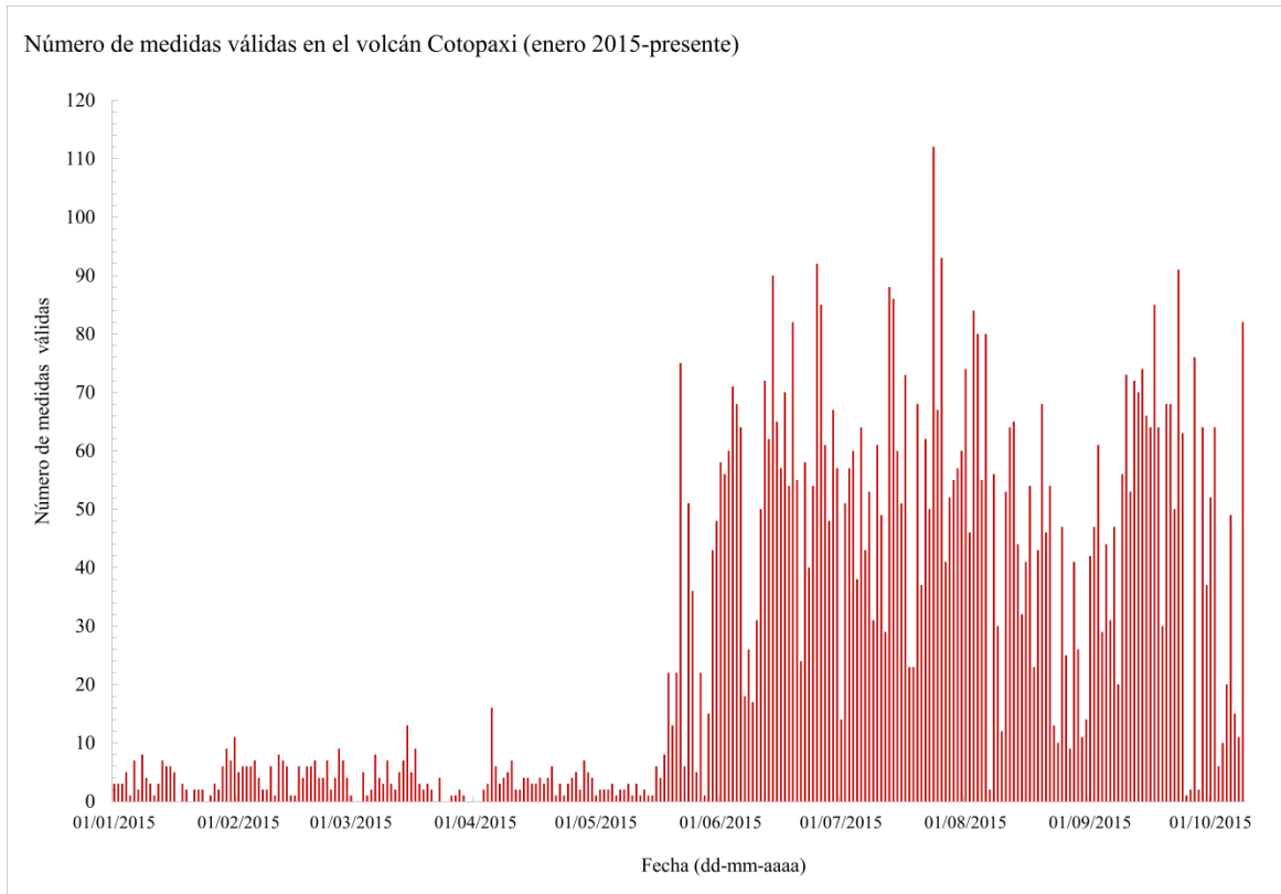
Fig. 3. Representación del número de medidas válidas en asociación con el flujo de SO_2 máximo diario - registradas en volcán Cotopaxi, desde enero 2015 al 9 de octubre del 2015.
