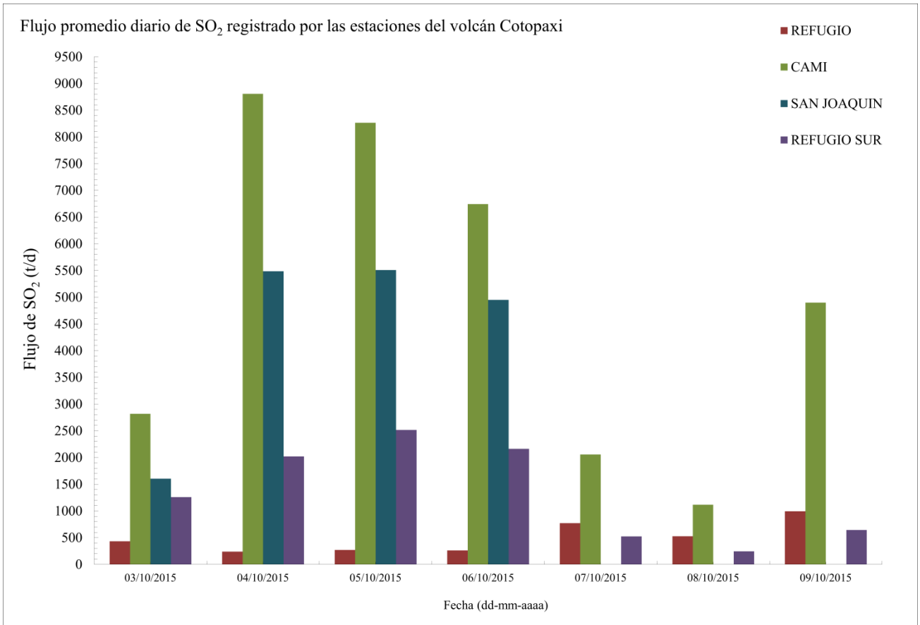
Fig. 1. Representación del flujo promedio diario de SO 2 , registrado por todas las estaciones del volcán Cotopaxi, para la 3 al 9 de octubre del 2015.
