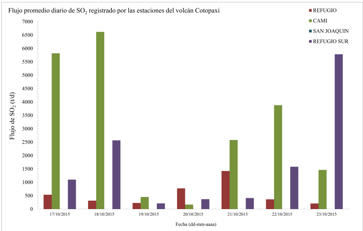
Fig. 1. Representación del flujo promedio diario de SO 2 , registrado por todas las estaciones del volcán Cotopaxi, para la 17 al 23 de octubre del 2015.
