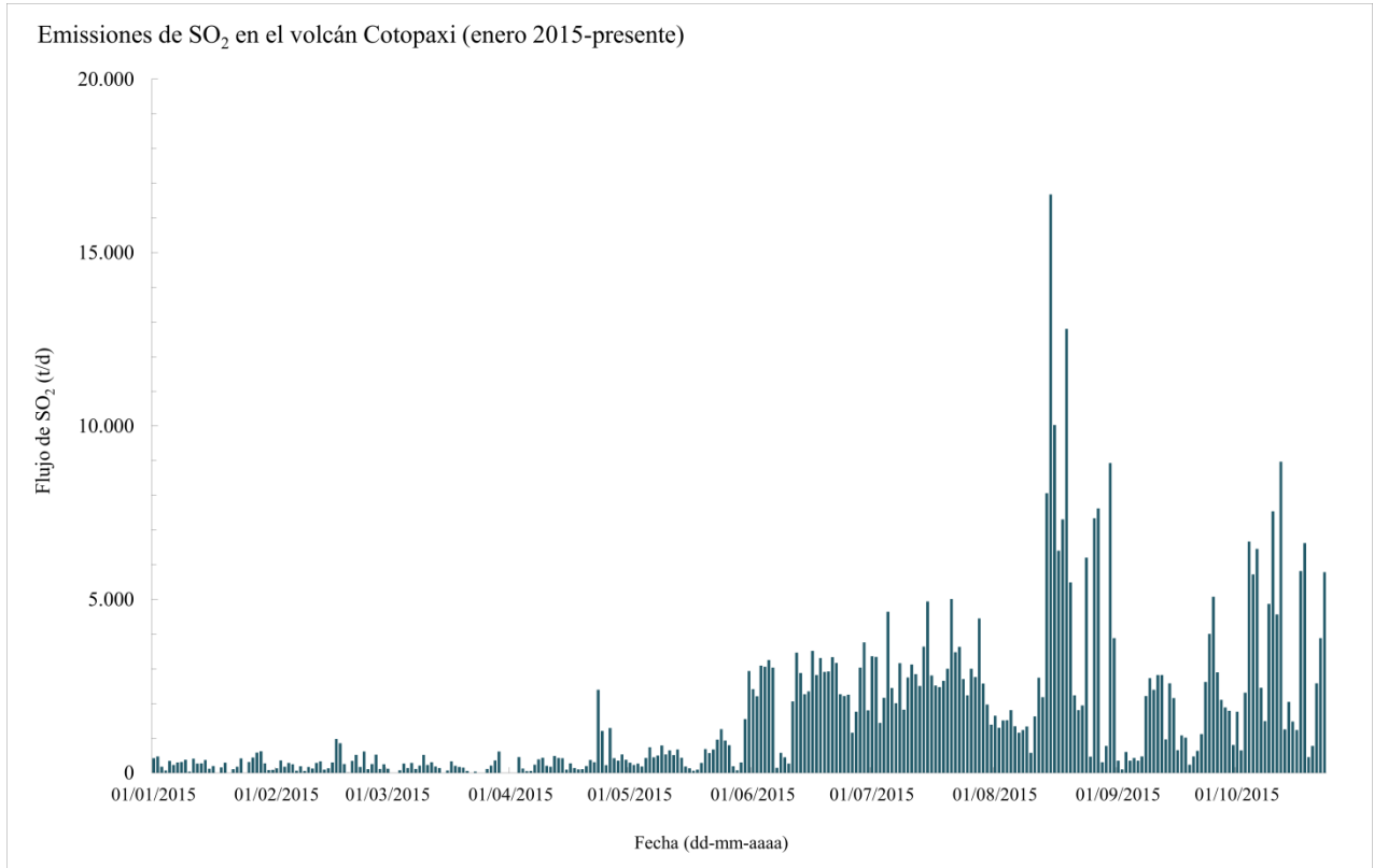
Fig. 2. Representación del máximo promedio diario flujo de SO_2 entre todas las estaciones permanentes del volcán Cotopaxi desde enero 2015 al 23 de octubre del 2015.
