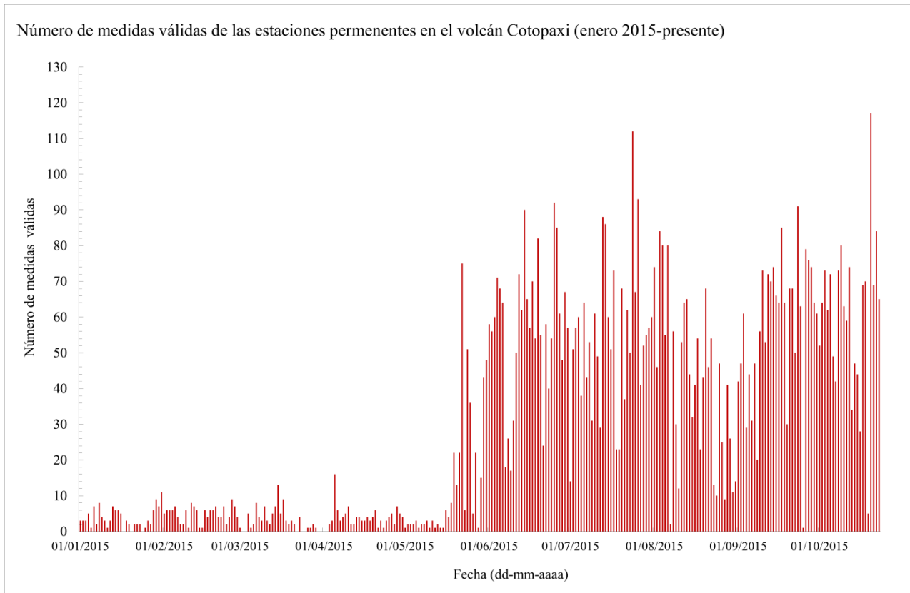
Fig. 3. Representación del número de medidas válidas en asociación con el flujo de SO_2 máximo diario - registradas en volcán Cotopaxi, desde enero 2015 al 23 de octubre del 2015.
