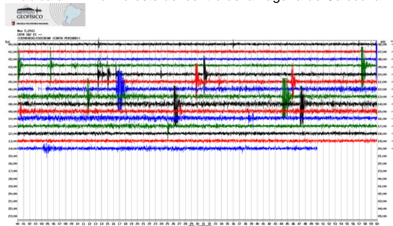
Figura no.2 Registro sísmico de la estación COTA del día 2 de noviembre de 2011. La estación COTA se ubica a 4 km al noreste del centro de la Laguna de Cuicocha
