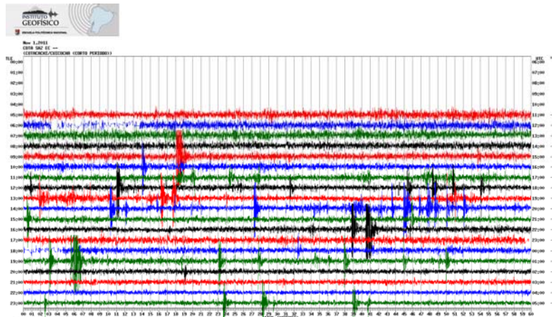
Figura no.1 Registro sísmico de la estación COTA del día 1 de noviembre de 2011. La estación COTA se ubica a 4 km al noreste del centro de la Laguna de Cuicocha
