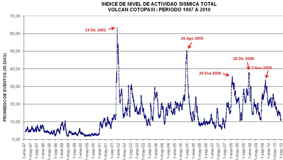
Figura 1. Índice de actividad sísmica del volcán Cotopaxi. Se observa baja actividad con tendencia descendente.
