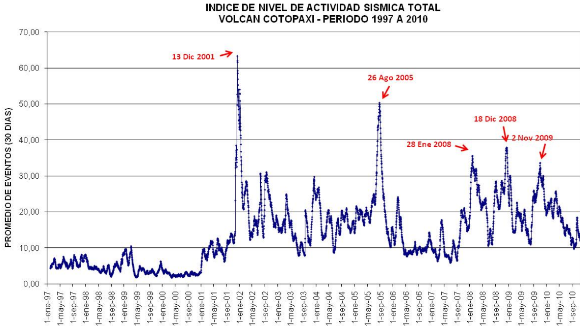
Figura 1. Índice de actividad sísmica del volcán Cotopaxi. Se observa baja actividad con tendencia descendente.
